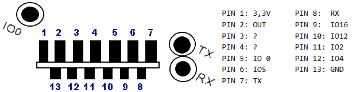
Bild: 8 - Unterseite schematisch
