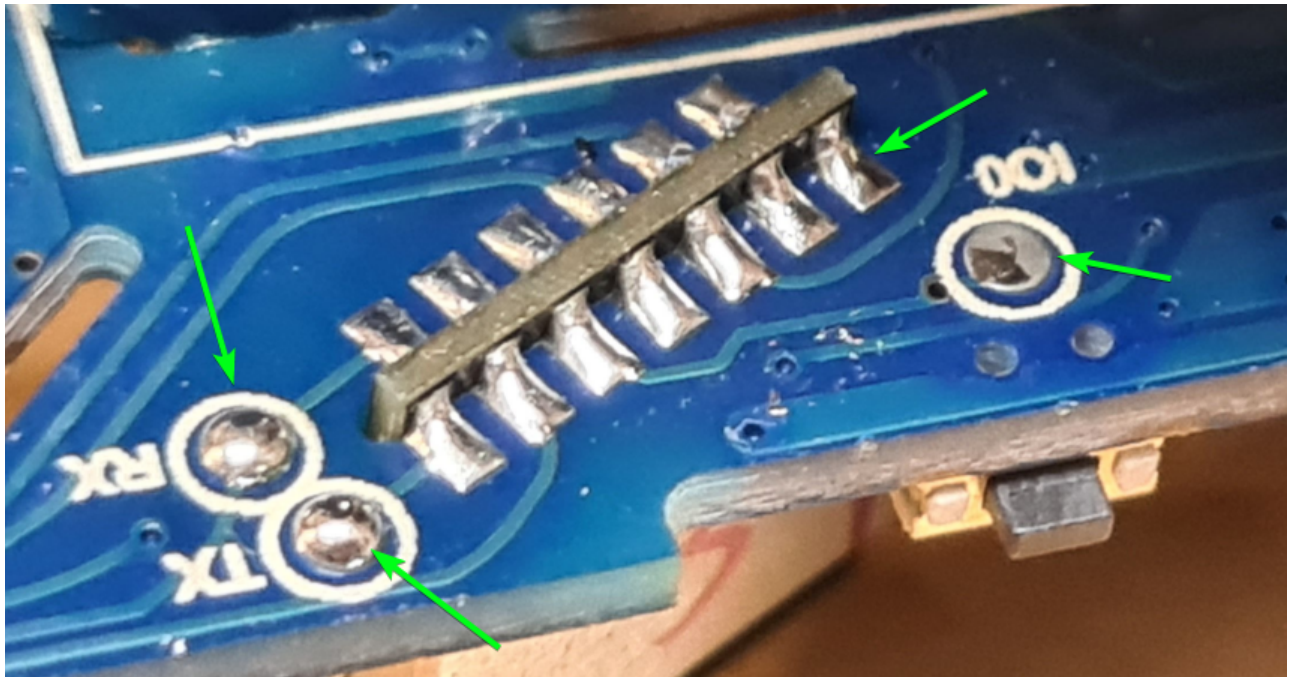
PIN-Belegung
