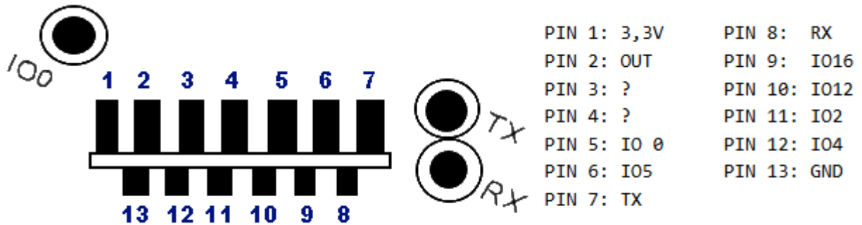
Bild: 8 - Unterseite schematisch
