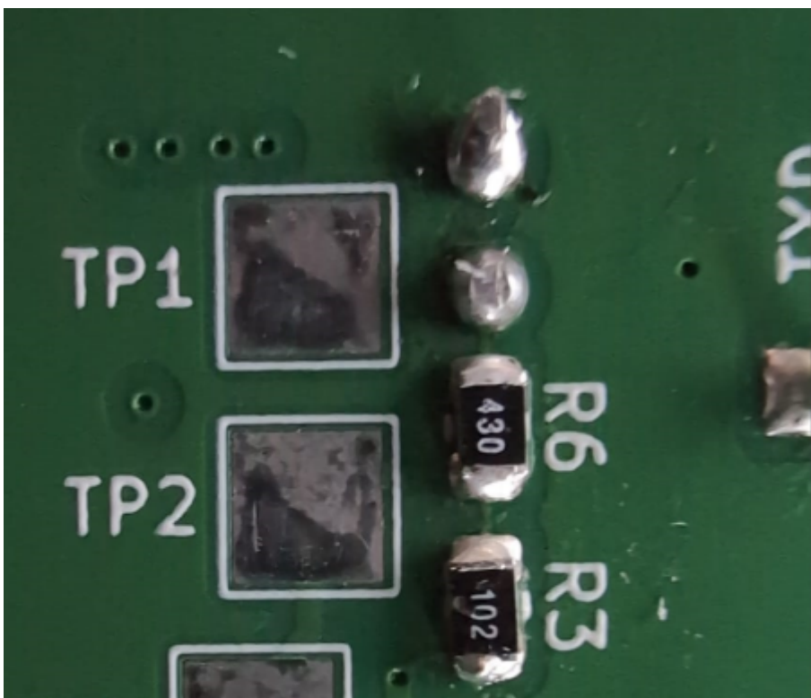
Widerstände des Spannungsreglers (5.1V)
